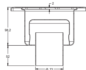
Ø 70 BOTTOM OUT - 20x20 cm
