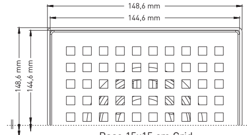
Base 15x15 cm Grid
