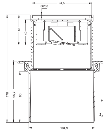
Ø 100 Bottom Out
