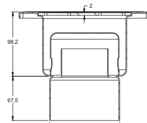
Ø 100 BOTTOM OUT - 20x20 cm
