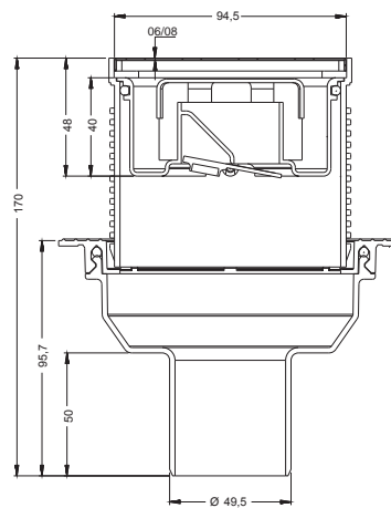
Ø 40 - Ø 50 Bottom Out
